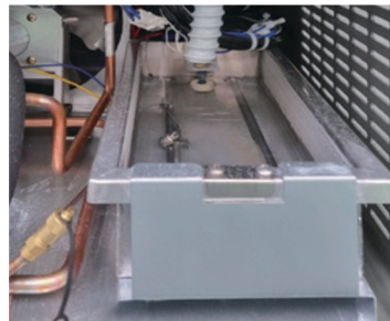
제상수 자연 증발장치 Defrosting water natural evaporation
